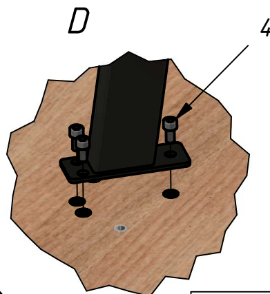
Схема сборки КС - 60
